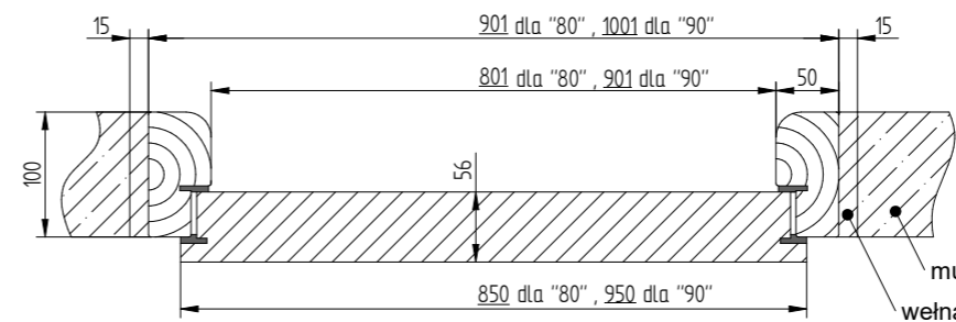
ECO-POŻ EI30 przekrój poziomy
