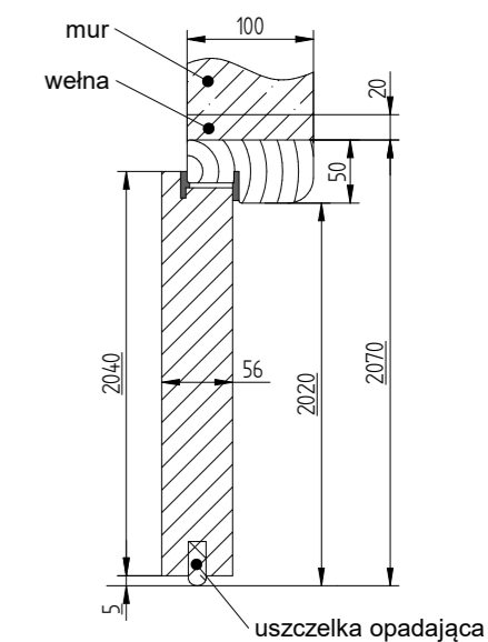
ECO-POŻ EI30 przekrój pionowy
