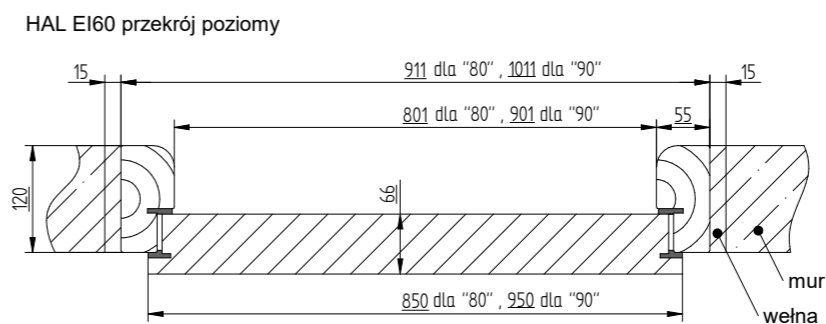
przekrój ościeżnicy do HAL EI30 i HAL EI60
