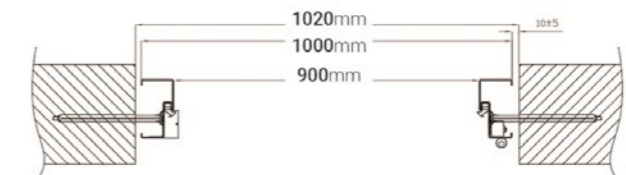
PRZYBLIŻONY WYMIAR OTWORU MONTAŻOWEGO
